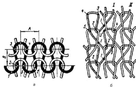
Рис. 1. Схема будови петель трикотажу: а – поперечнов'язана петля; б – основнов'язана петля.
